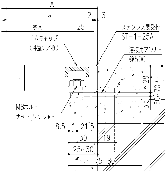
断面詳細図
