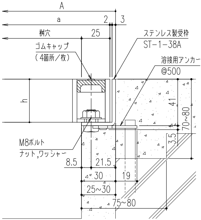
断面詳細図
