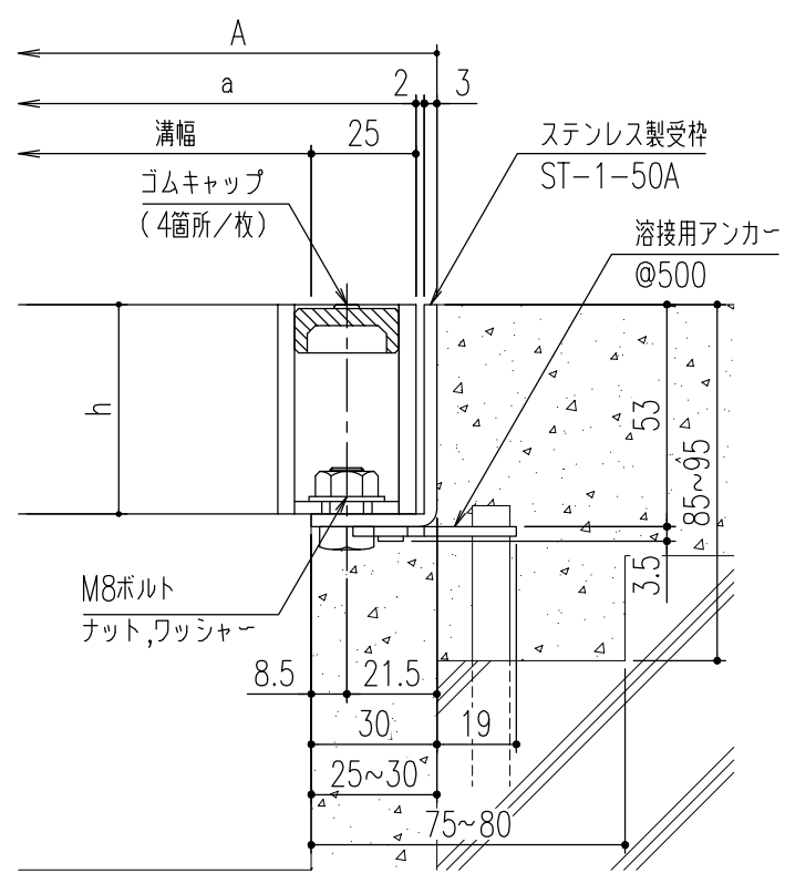
断面詳細図
