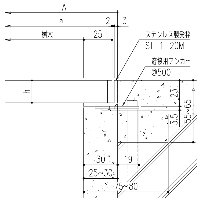
断面詳細図
