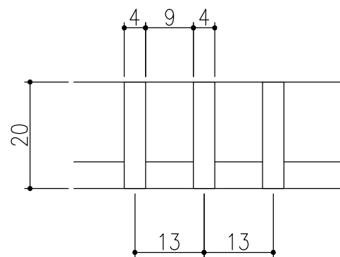
フラットバー詳細図
