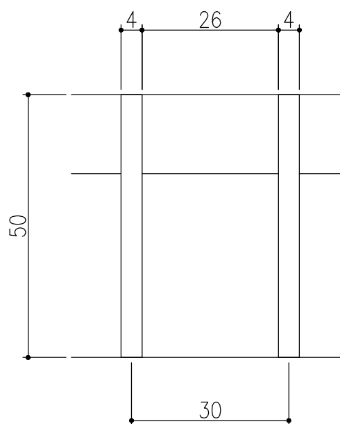
フラットバー詳細図
