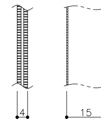
フラットバー詳細図
