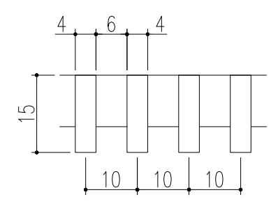
フラットバー詳細図
