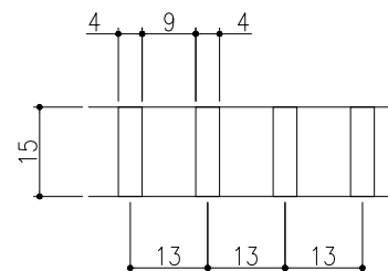
フラットバー詳細図
