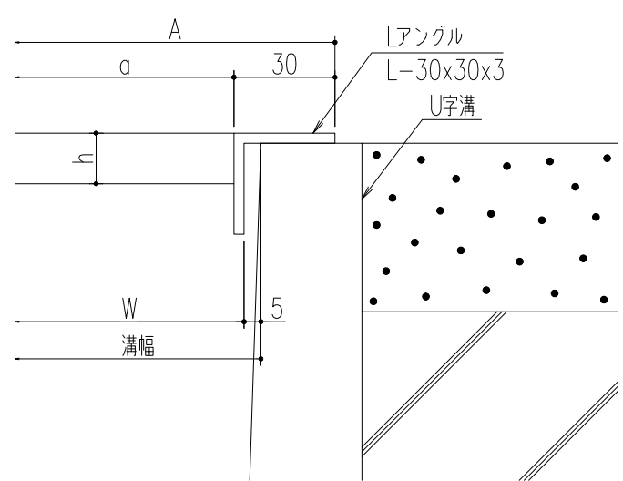
断面詳細図
