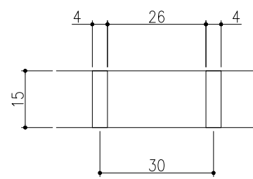
フラットバー詳細図
