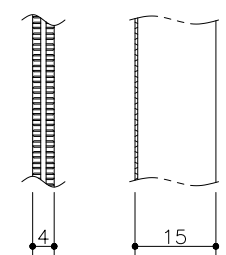
フラットバー詳細図
