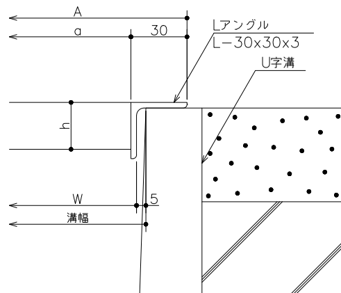
断面詳細図
