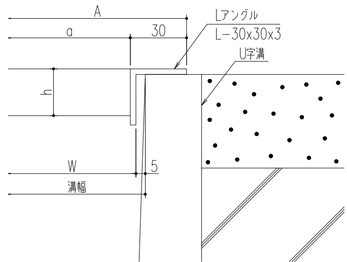
断面詳細図
