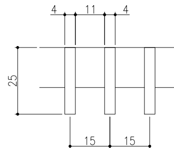
フラットバー詳細図
