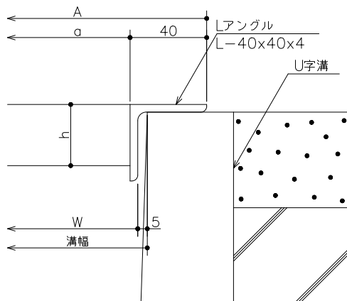
断面詳細図
