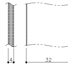
フラットバー詳細図
