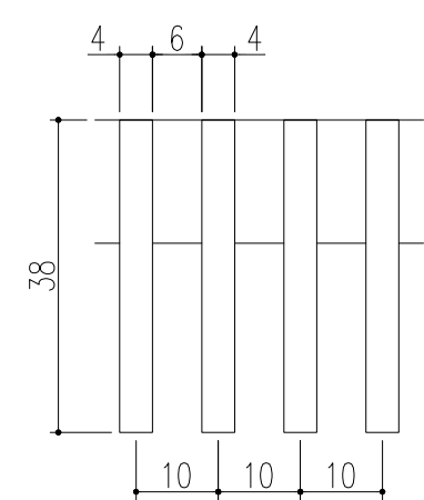
フラットバー詳細図
