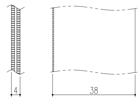
フラットバー詳細図
