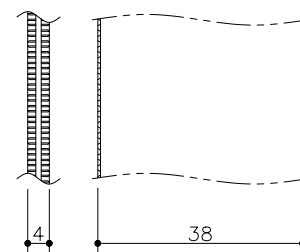
フラットバー詳細図
