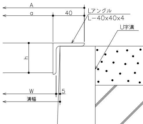
断面詳細図
