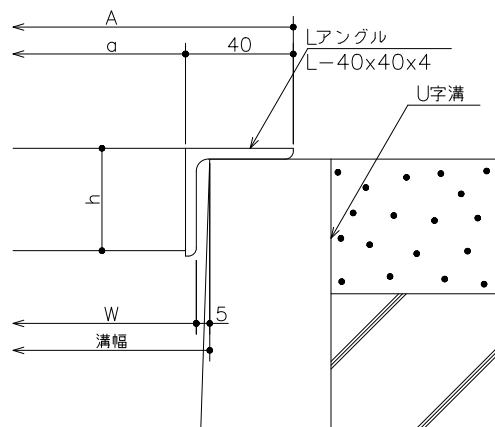
断面詳細図
