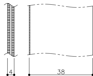
フラットバー詳細図
