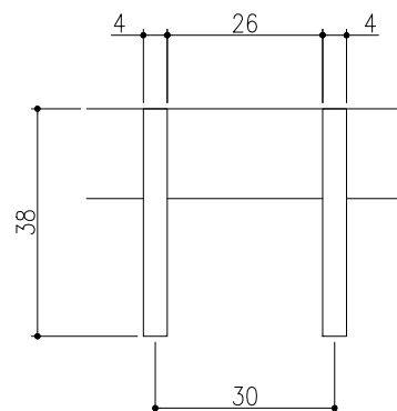
フラットバー詳細図
