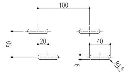
排水穴形状
