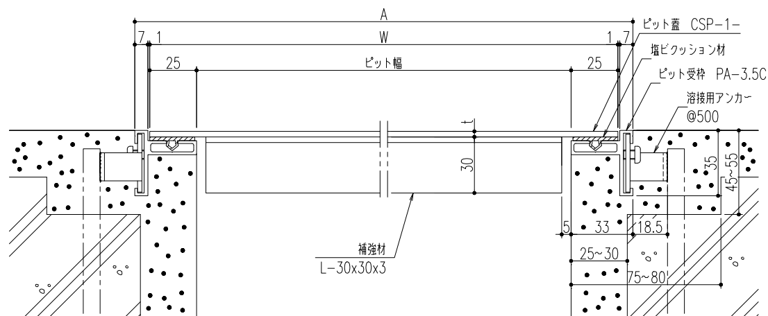
断面詳細図 S=1/2
