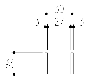
ベアリングバー 詳細図
