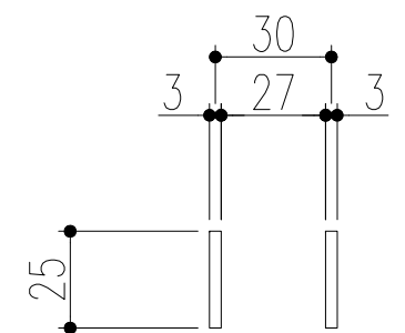
ベアリングバー 詳細図
