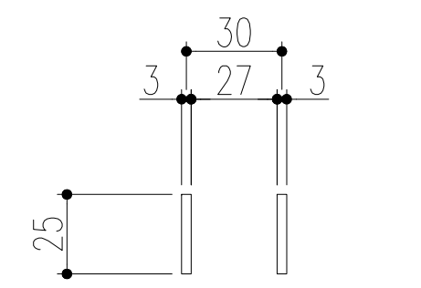
ベアリングバー 詳細図
