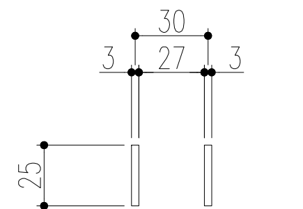
ベアリングバー 詳細図
