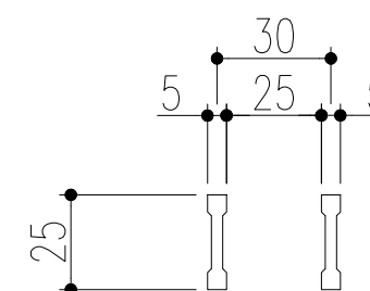
ベアリングバー 詳細図
