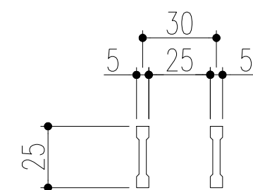
ベアリングバー 詳細図
