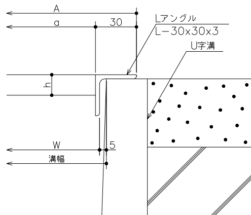
断面詳細図
