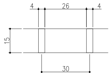
フラットバー詳細図
