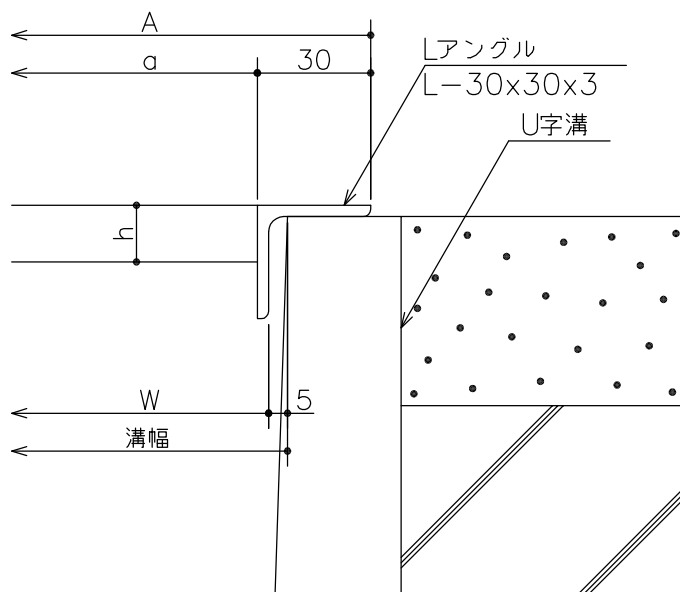
断面詳細図
