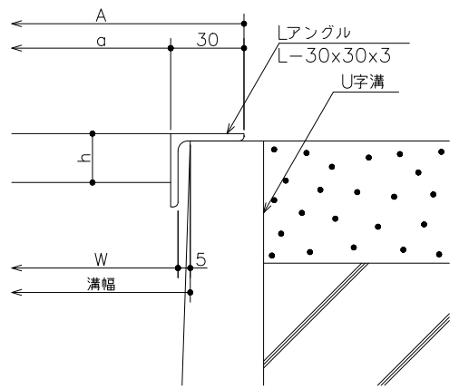
断面詳細図
