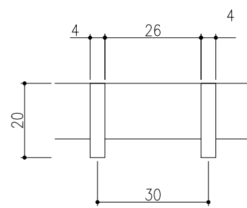
フラットバー詳細図
