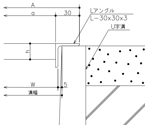
断面詳細図
