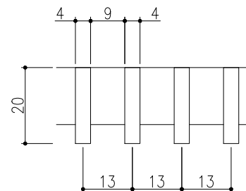
フラットバー詳細図
