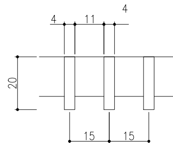
フラットバー詳細図
