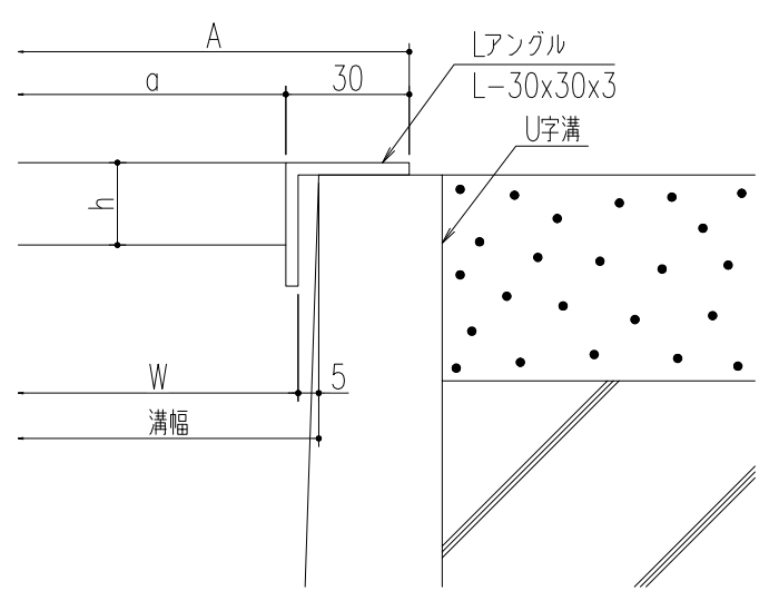
断面詳細図
