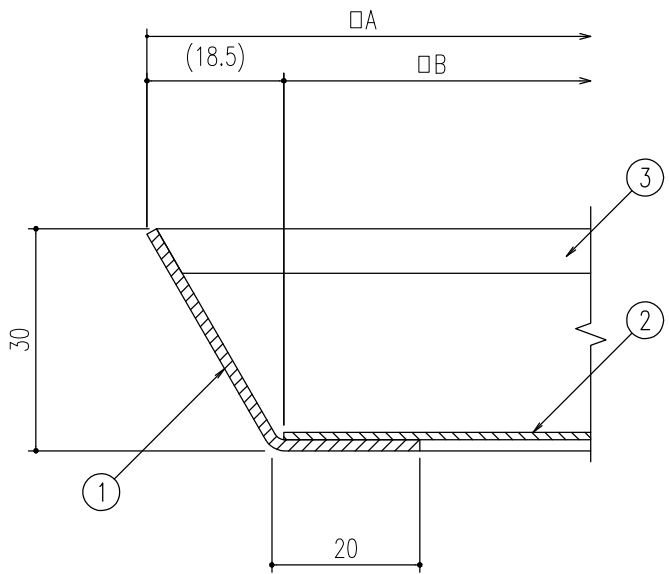
拡大詳細図 S=1/1
