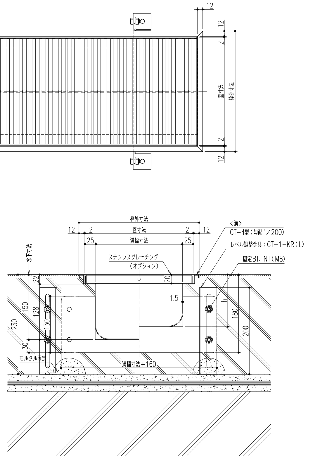
クリーントラフ<溝><上樹><下樹> 主材質;t=1.5 SUS304 2B 表面処理;目地部HL仕上 その他;SUS304 2B
