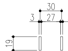
ベアリングバー 詳細図
