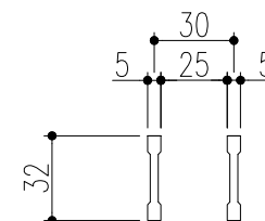
ベアリングバー 詳細図
