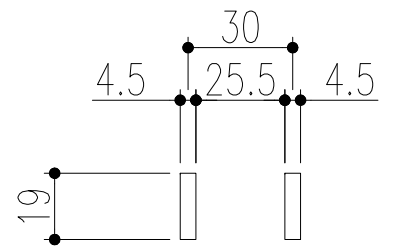
ベアリングバー 詳細図
