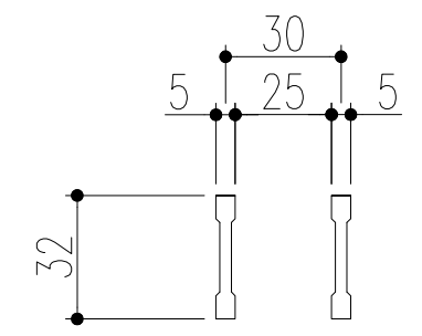
ベアリングバー 詳細図
