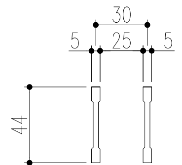
ベアリングバー 詳細図
