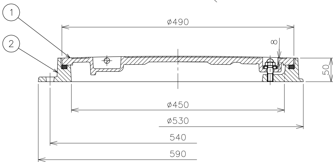
A-A断面
