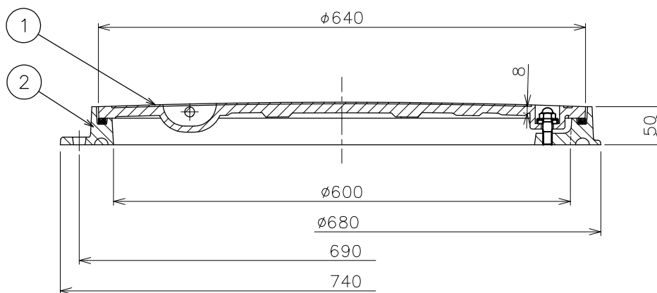
A-A断面
