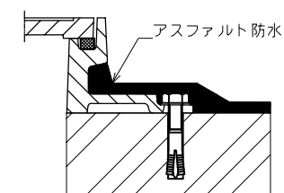
アスファルト防水納まり例
