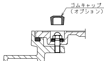
ボルト部納まり図
