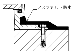
アスファルト防水納まり例
