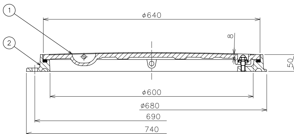
A-A断面
