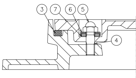
ボルト固定部詳細図 (1/3)
