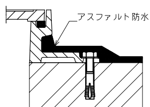
アスファルト防水納まり例
