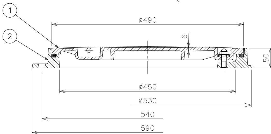
A-A断面
