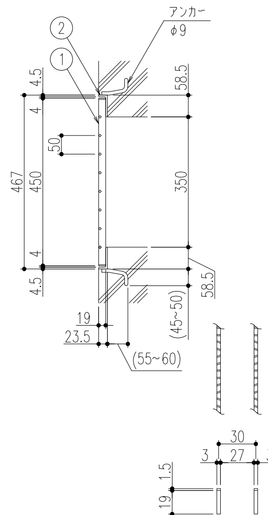
ベアリングバー 詳細図
