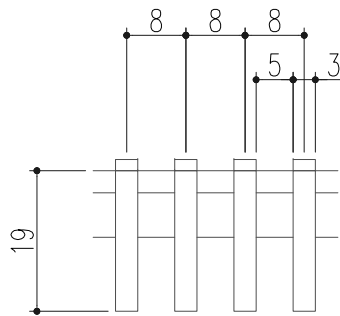
ベアリングバーの断面詳細図
