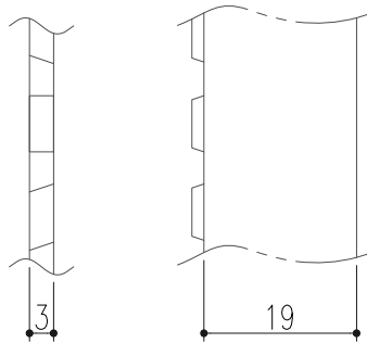
ベアリングバーの詳細図
