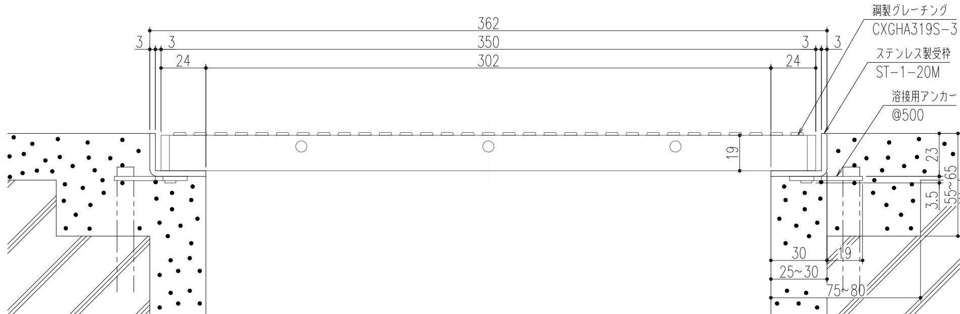
断面詳細図 S=1/2
