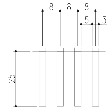
ベアリングバーの断面詳細図
