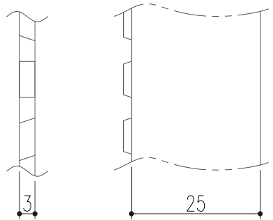
ベアリングバーの詳細図
