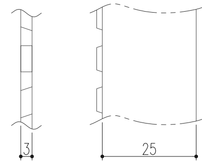
ベアリングバーの詳細図
