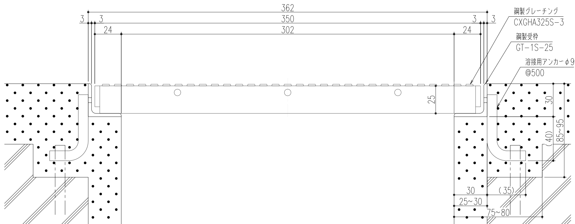
断面詳細図 S=1/2
