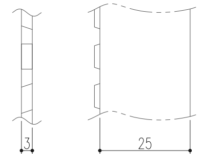
ベアリングバーの詳細図
