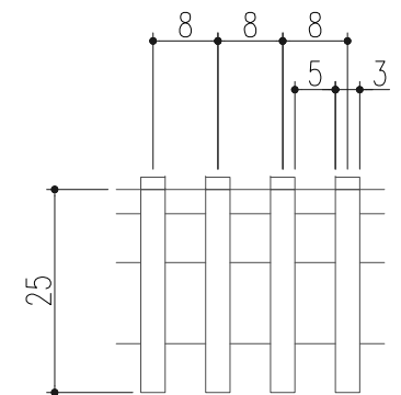
ベアリングバーの断面詳細図
