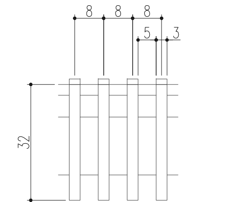
ベアリングバーの断面詳細図
