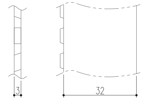
ベアリングバーの詳細図
