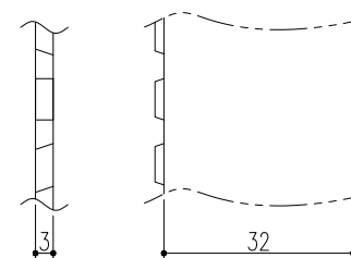
ベアリングバーの詳細図
