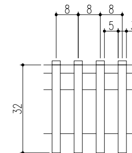
ベアリングバーの断面詳細図
