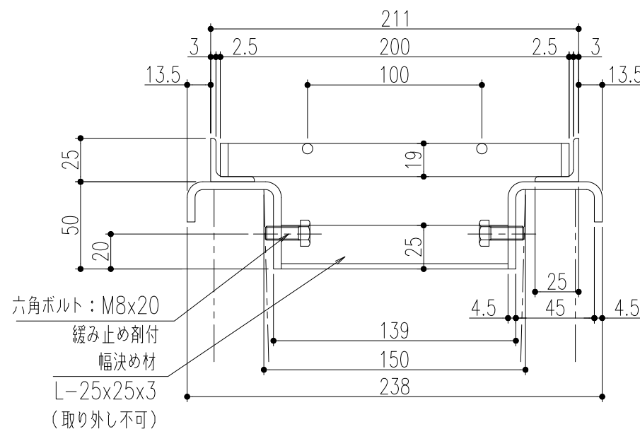
断面詳細図 S=1/3
