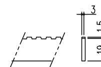
ベアリングバー 詳細図
