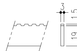
ベアリングバー 詳細図
