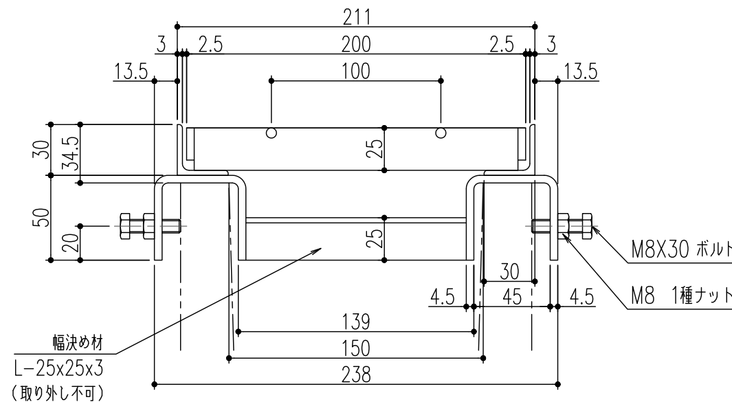
断面詳細図 S=1/3
