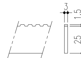
ベアリングバー 詳細図
