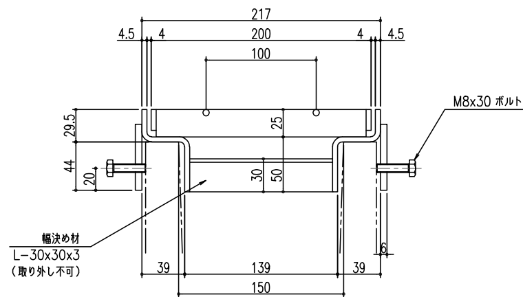
断面詳細図 S= 1/3
