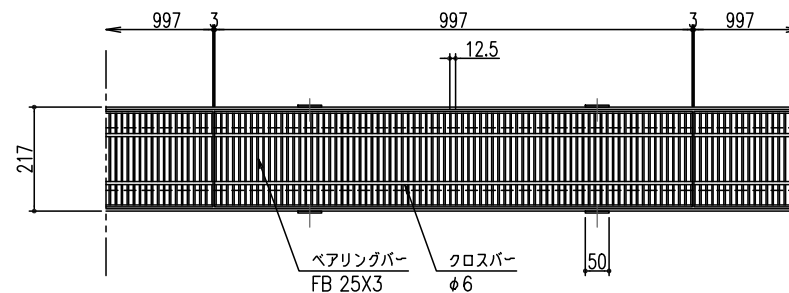
平面詳細図 S= 1/10
